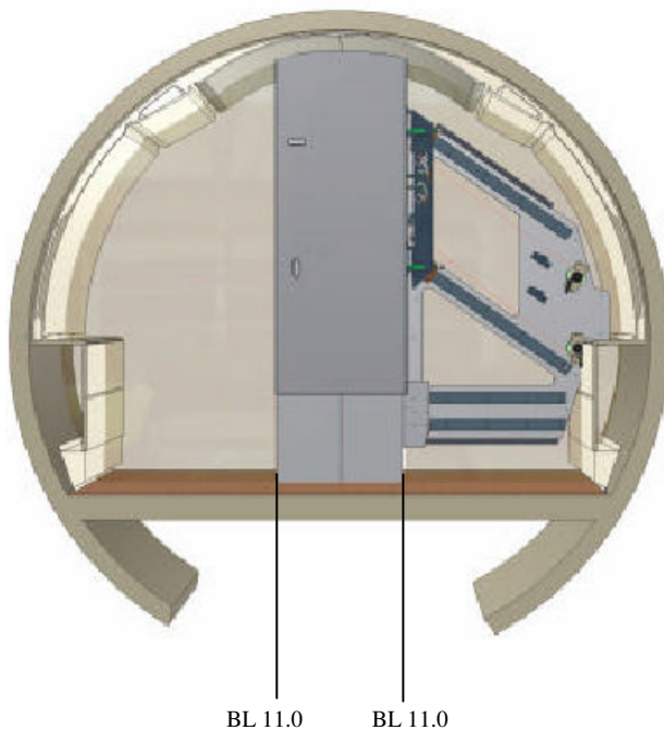
3519-138-3 MANUAL DOOR SHOWN
