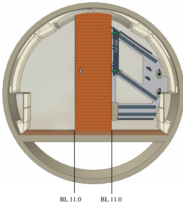
3519-137-3 MANUAL DOOR SHOWN
