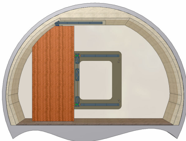
3519-105-1 Door SHOWN
